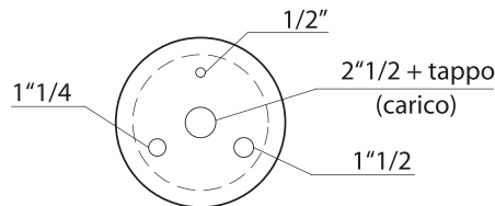
particolare boccaporto
